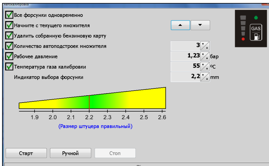
Рис. 27 Окно «Автокалибровка».
